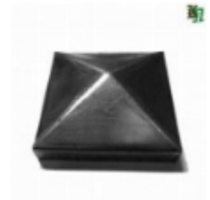
Заглушка на столб 50x50, арт. 15.054.02 50x50x1мм Вес: 0.036 кг Цена: 11 руб.
