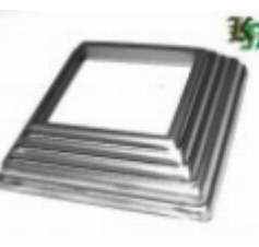
Основание блясины, арт. 13.360.02 100x100x1мм, кв.60x60мм Вес: 0.09 кг Цена: 37 руб.
