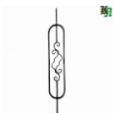
Балясина с художественным узором, арт. 3083 1000х160мм, кв.12х12мм,полоса 6х12 Вес: 2.82 кг Цена (за шт): 640 руб.
