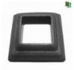
Основание блясины, арт. 7.1155 60x60мм, кв.30x30мм Вес: 0.09 кг Цена: 50 руб.
