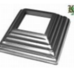
Основание блясины, арт. 13.350.02 100x100x1мм, кв.50x50мм Вес: 0.08 кг Цена: 37 руб.
