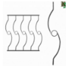
Балясина, арт. 3093 1000х150мм, кв.12х12мм Вес: 1.4 кг Цена (за шт): 470 руб.
