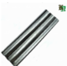
Обжимка, арт. 015201 1250x15x0,8мм Вес: 0.09 кг Цена (за штуку): 39 руб.
