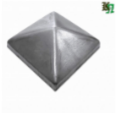
Заглушка на столб 60x60, арт. 15.055.36 60x60x1мм Вес: 0.03 кг Цена: 22 руб.
