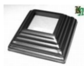
Основание блясины, арт. 13.319.01 80x80x1мм, кв.30x30мм Вес: 0.066 кг Цена: 38 руб.
