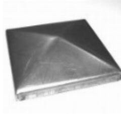
Заглушка, арт. 15.056 80x80x1мм Вес: 0.076 кг Цена: 25 руб.
