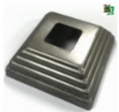
Основание блясины, арт. R10436.02 80x80x1мм, кв.25x25мм Вес: 0.075 кг Цена (за шт): 10 руб.
