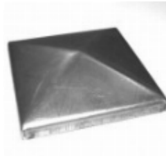
Заглушка, арт. 15.055 60x60x1мм Вес: 0.048 кг Цена (за шт): 22 руб.
