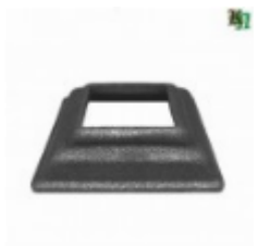
Основание блясины, арт. 7.321 80x80мм, кв.40x40мм Вес: 0.14 кг Цена: 85 руб.
