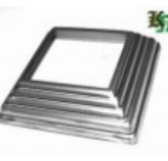
Основание блясины, арт. 13.360.01 100x100x1мм, кв.60x60мм Вес: 0.07 кг Цена: 45 руб.
