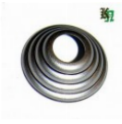
Основание балясины, арт. 13.348.01 д=50x1мм, отв.д=17мм Вес: 0.02 кг Цена: 11 руб.
