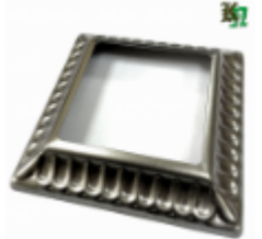
Основание балясины штампованное, арт. 8.879 170x170x1 кв. 100x100 Вес: 0.19 кг Цена (за шт): 150 руб.
