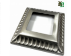
Основание блясины штампованное, арт. 8.881 170x170x1 кв. 80x80 Вес: 0.21 кг Цена (за шт): 150 руб.
